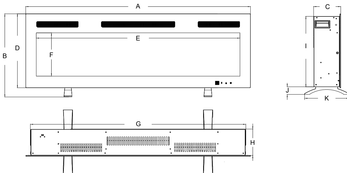
Dimensiones del producto (mm)
