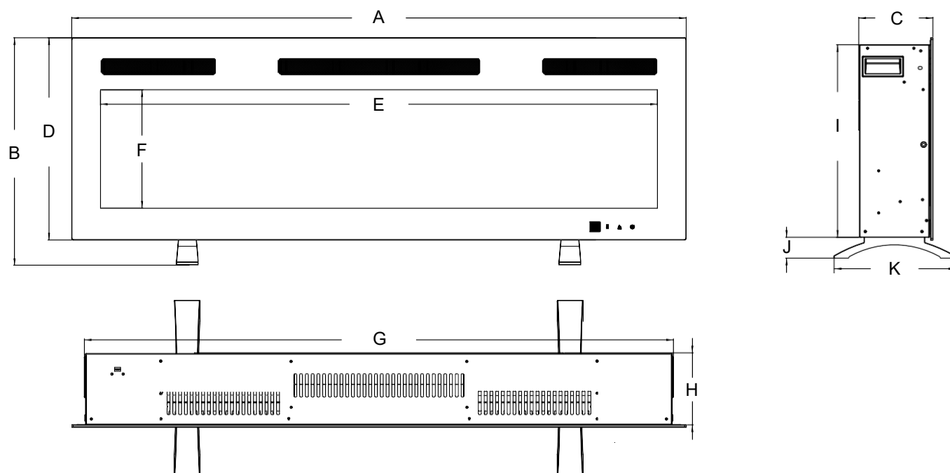
Dimensioni del prodotto (mm)
